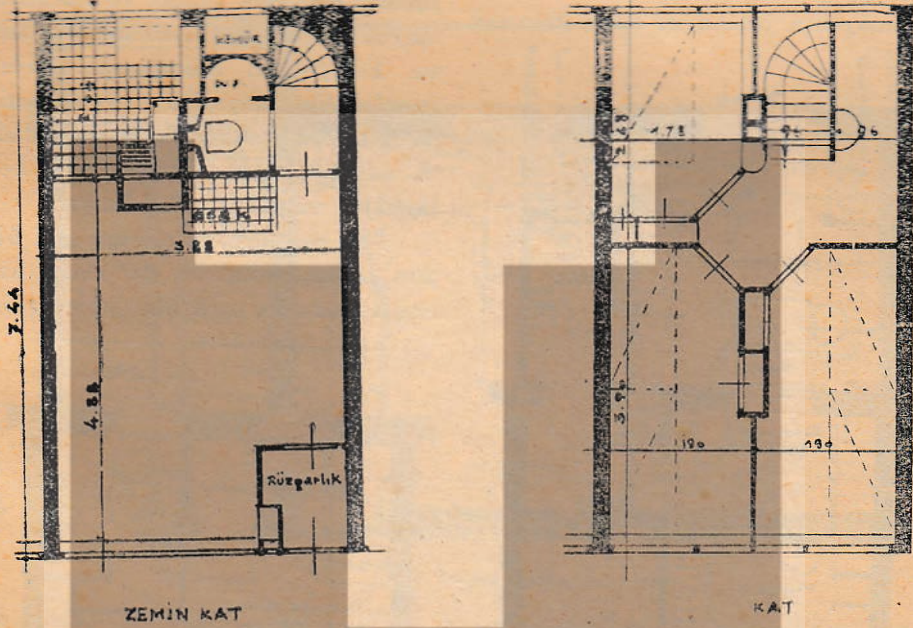
1926 da Rotterdam'da yapılmış iki katlı sıra evlerden bir örnek. İnşaat sahası 30,50 metre karedir. Ucuza mal olması için fabrikada hazırlanmış hafif beton kirişler kullanılmıştır.
